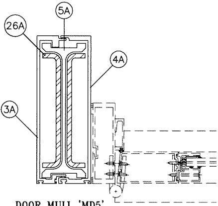
DOOR MULL 'MD5'
