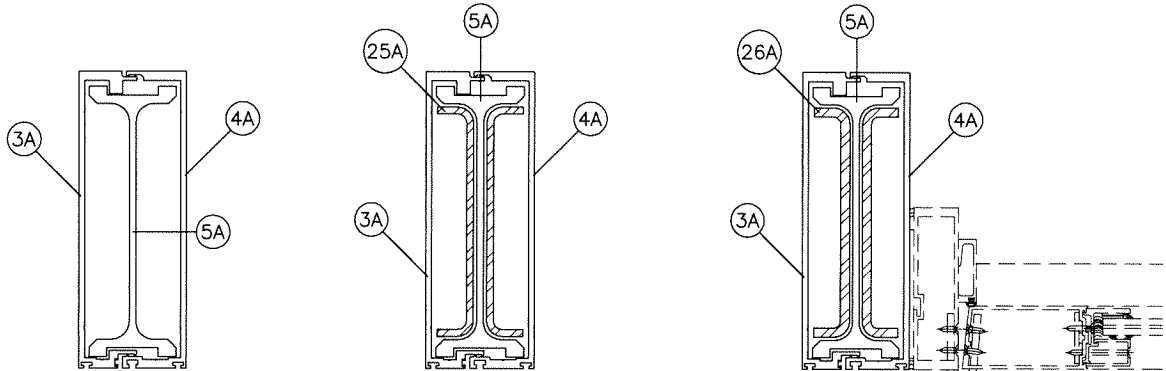
DOOR MULL 'MD3'
